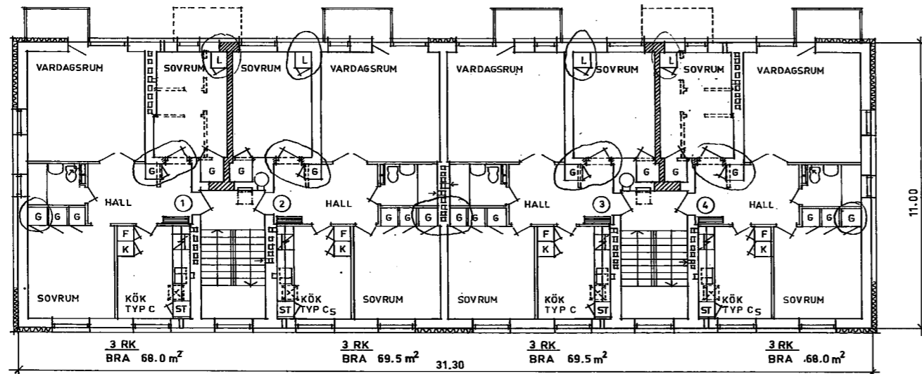
VÅNINGSPÅN 1-3.
